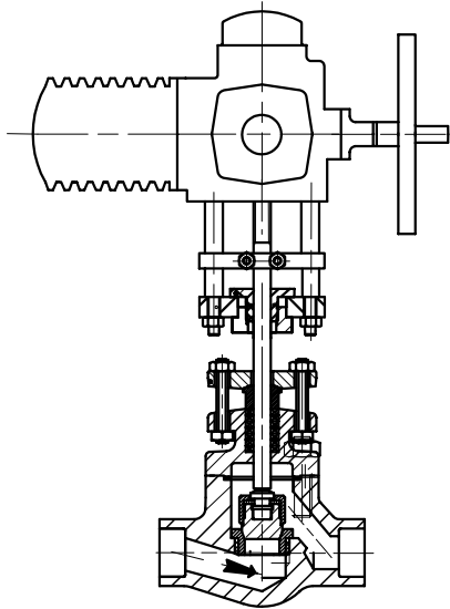
MOTORISATION ELECTRIQUE / ELECTRIC ACTUATOR
