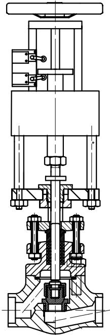
MOTORISATION PNEUMATIQUE / PNEUMATIC ACTUATOR
