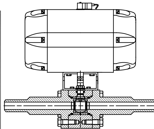
MOTORISATION PNEUMATIQUE / PNEUMATIC ACTUATOR
