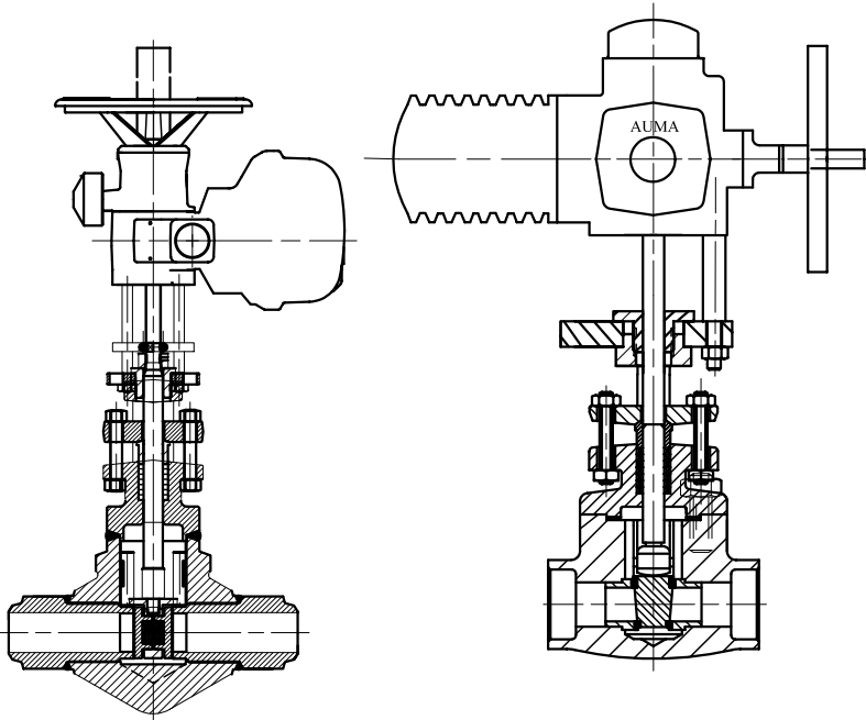
MOTORISATION ELECTRIQUE / ELECTRIC ACTUATOR
