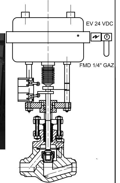
MOTORISATION PNEUMATIQUE / PNEUMATIC ACTUATOR
