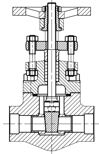
SOCKET WELD END SUIVANT/ acc. to ANSI B16-11
